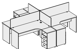
841PRx2/841Lx2/842x4/877x2/874x2 - 3825x2405x750(1150)
