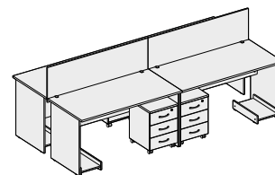
810x4/817x4/878x4/877x2 - 2800x1425x750(1150)
