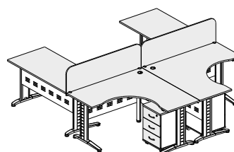
441.04-Mx2/410-Mx2/177x2/117x2 - 2825x2800x750(1150)
